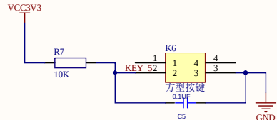
按键电路
