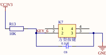
按键电路
