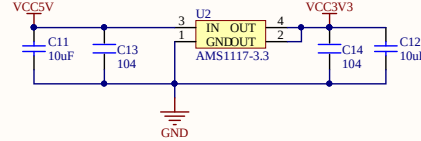
降压电路
