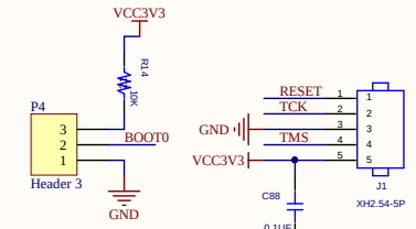
BOOT0开关
